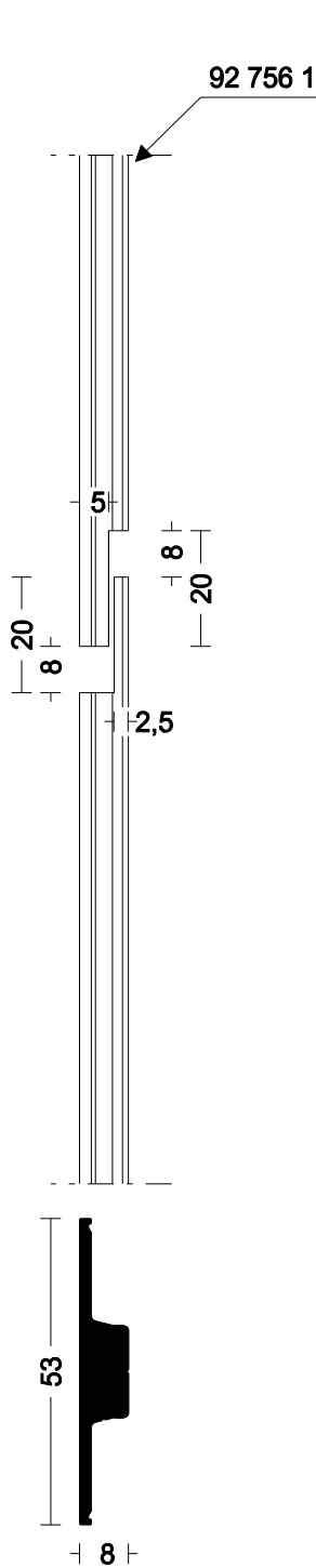
Ausklinkung SG-Andruckprofil
